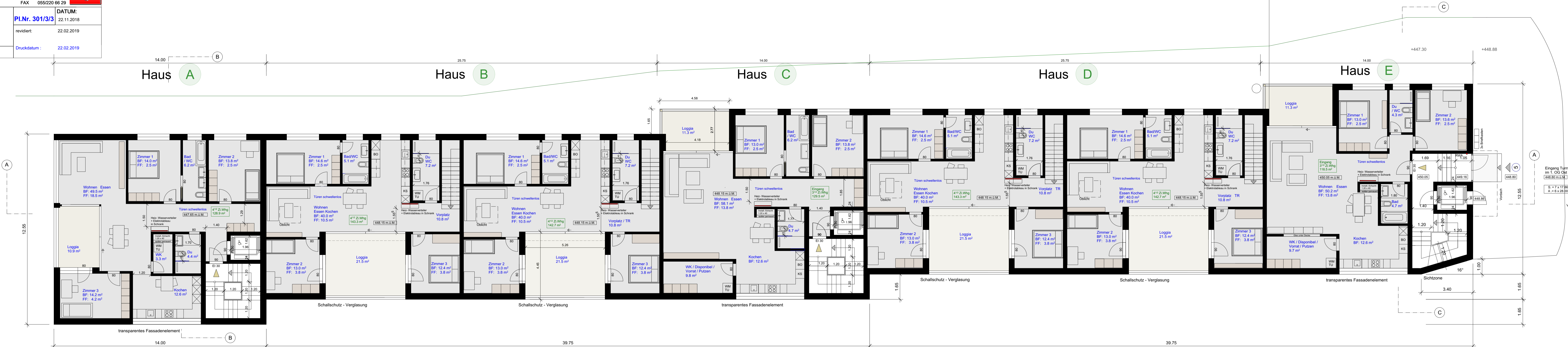
Grundriss 1. Obergeschoss Mst. 1:100
