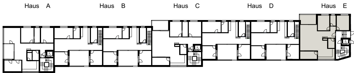
Grundriss 1. Obergeschoss 1:600
